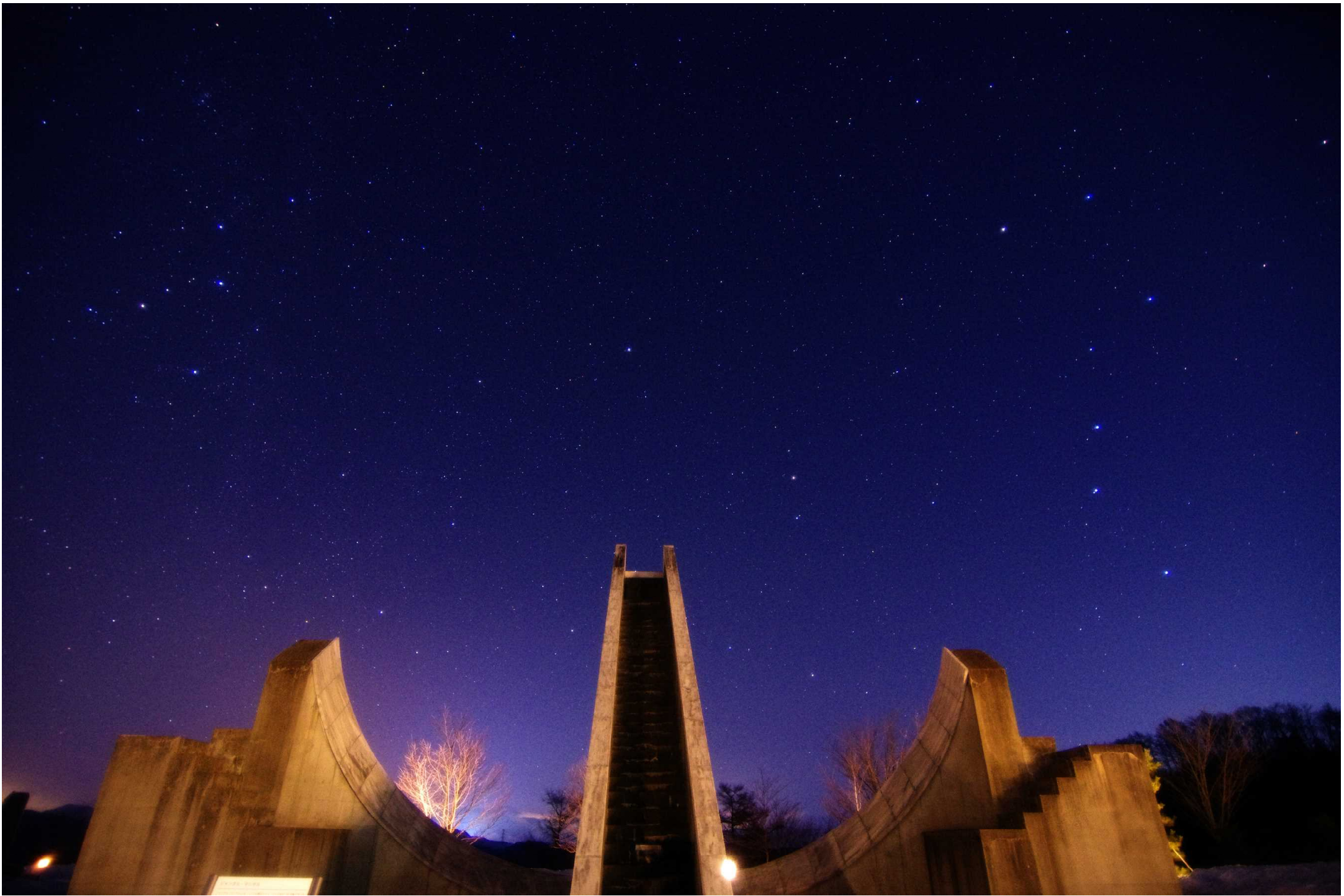
図1 北斗七星、カシオペヤ座とモニュメント 2017.0224.19:53 出典：ぐんま天文台
