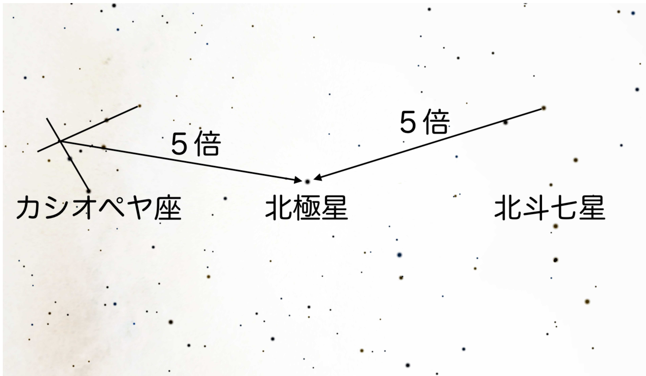
図2 北極星の探し方① 出典：ぐんま天文台
