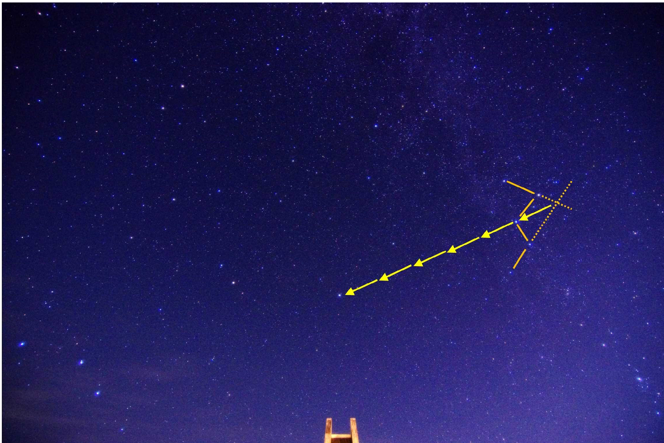
図3 北極星の探し方② 出典：ぐんま天文台
